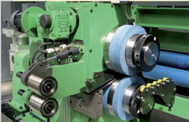
Кромкообрезные ножницы для самых разных материалов, толщин и ширины ленты (полотнища)
