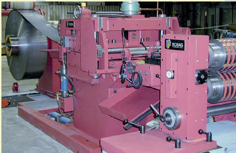
Комбинированное устройство наладки с поперечными вспомогательными ножницами
