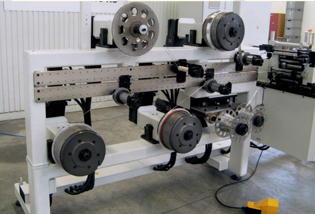
Gesamtansicht Wickleinheiten mit individuell verstellbaren Elementen General view of recoiling system including individually adjustable elements
