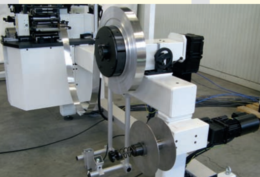
Abwickelhaspel ausgelegt für Schlaufenbetrieb und Direktabzug mit Papieraufwickler Decoiler laid out for loop and direct feeding mode including paper rewinder
