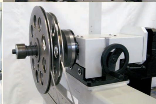
Wickeln auf Trommeln, Spulen, Kerne oder Kassetten mit einstellbaren Wickelzügen von 2-200 N oder im Friktionsverfahren für den Ø-Bereich von 76-600 mm Recoiling on drums, spools, cores or cassettes with adjustable retention from 2 to 200 N or by friction system for Ø range from 76 to 600 mm
