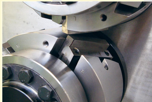
Coltelli regolabili per regolazione profondità di penetrazione e recupero dopo l'affilatura
